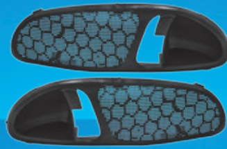
EK.0408 (LD - cinza antracite) EK.0409 (LE - cinza antracite) Moldura dianteira VW Gol G3
